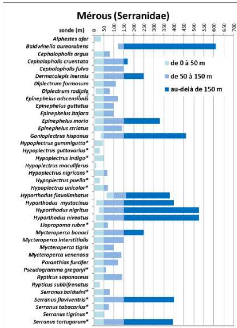
Figure 42. Distributions bathymétriques des mérours et autres Serranidae commerciaux signalés en Haïti
